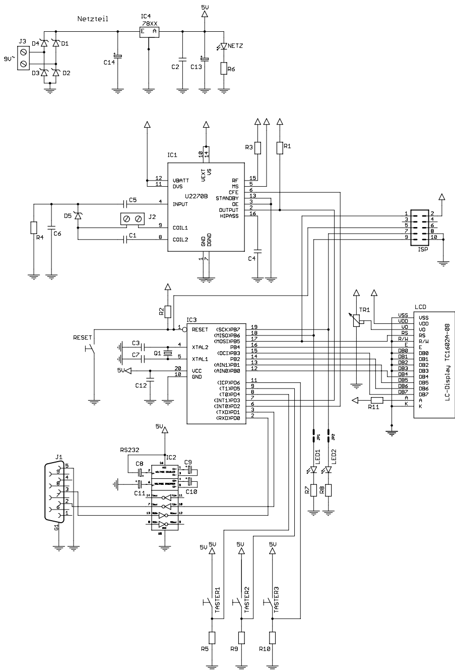
Schaltplan für den RFID-125kHz-Empfänger-Bausatz
