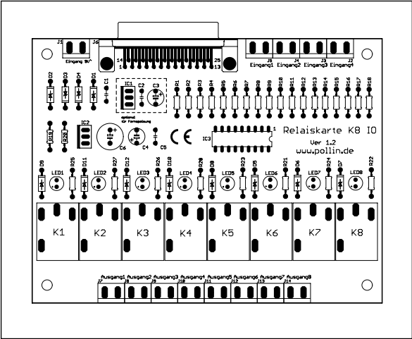
Bestückungsdruck PC-Relaiskarte K8 IO
