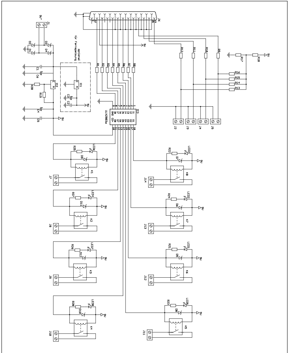
Schaltplan für die PC-Relaiskarte K8 IO
